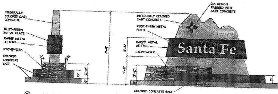
⑤ BACK ELEVATION SCALE: 3/8" = 1'-0"
